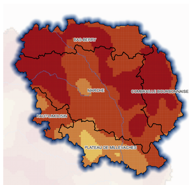
Densité de vaches viande au km² en 2010 (*)
