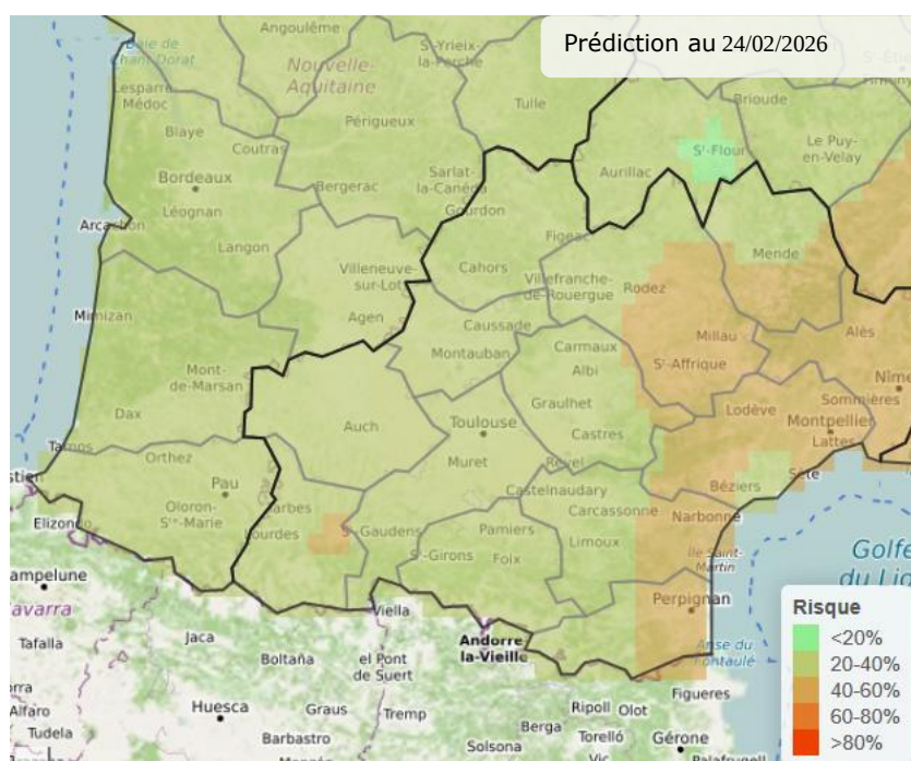
Figure 2 : évolution de la probabilité de captures du charançon de la tige du colza dans le Sud-Ouest. Ces prévisions de vol sont obtenues à partir de l'outil « Prédiction des vols de ravageurs »
