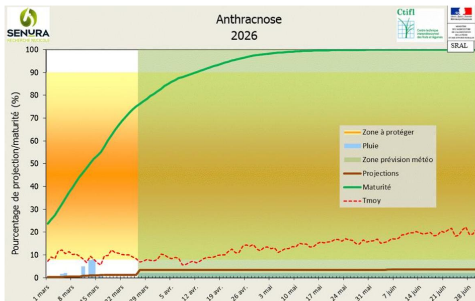
Figure 2. Modélisation INOKI des projections Antracnose à Gnomonia , secteur LA ROQUE (24).
