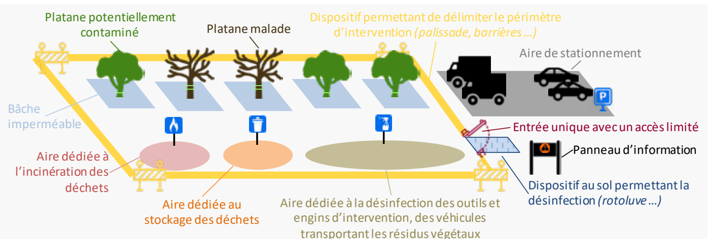
Fig. 13 - Configuration d'une aire de chantier d'abattage
